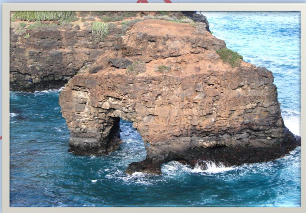
Roque horadado por cuevas por donde entra y sale el mar.
