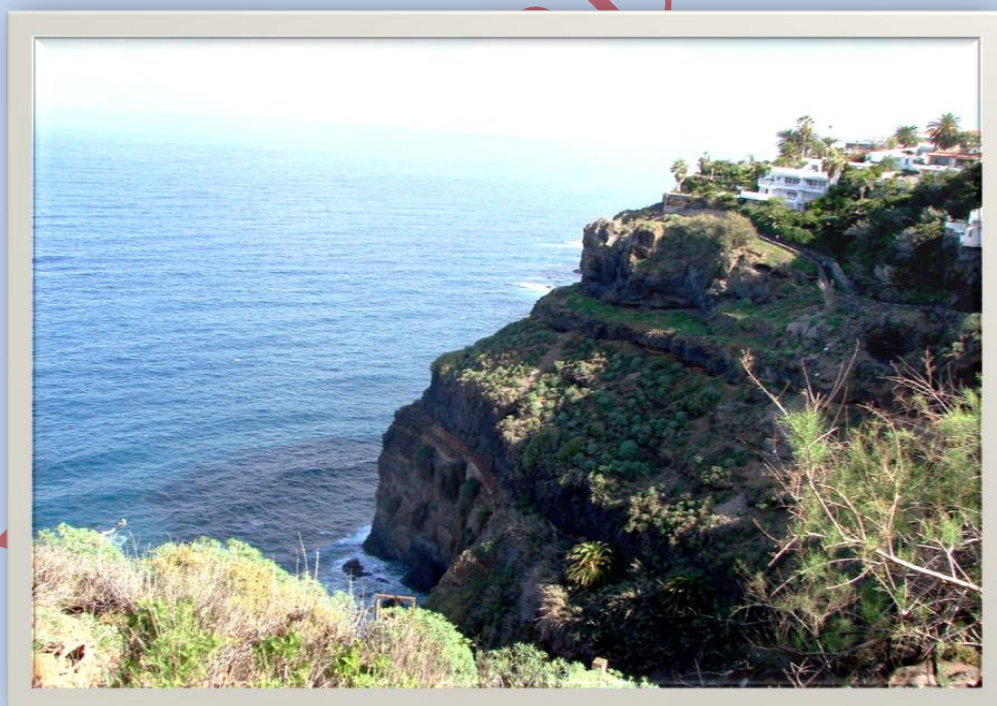
Pasado el barranco de La Fajana se pueden observar la costa acantilada del lugar.
