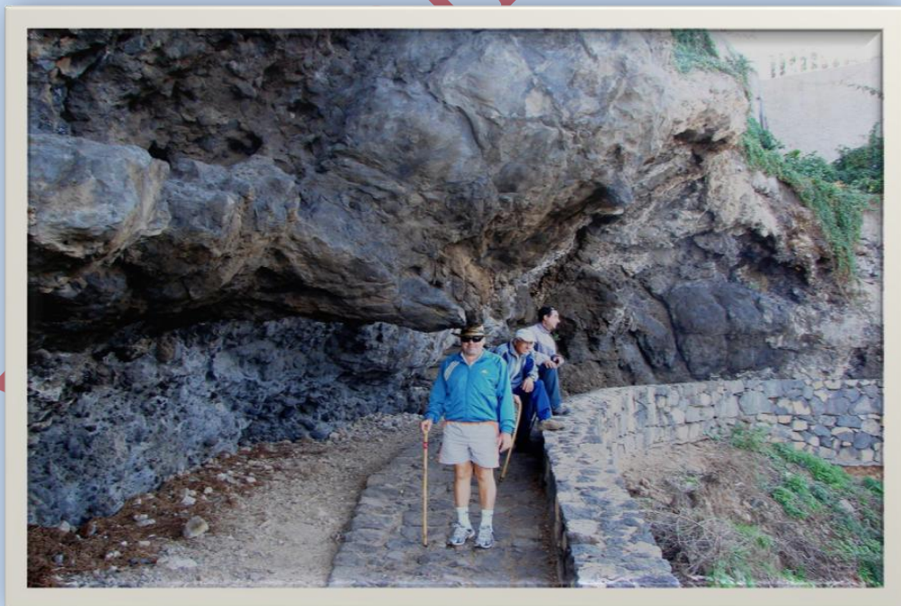
Tramo del sendero donde pasamos por debajo de formaciones de interés geológico y geomorfológico que nos indican el pasado volcánico de la zona, ¡ojo con la cabeza!
